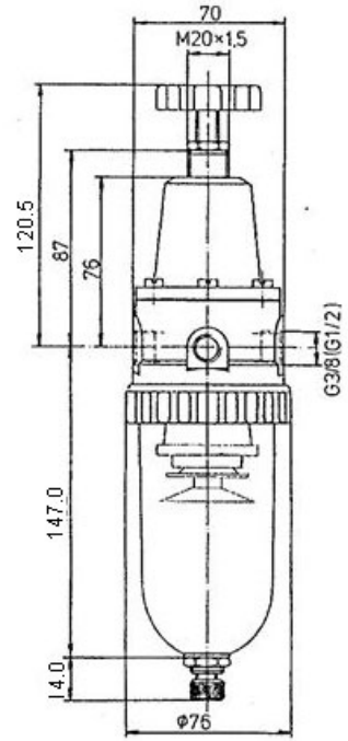
Filterregler mit Metallbehälter
