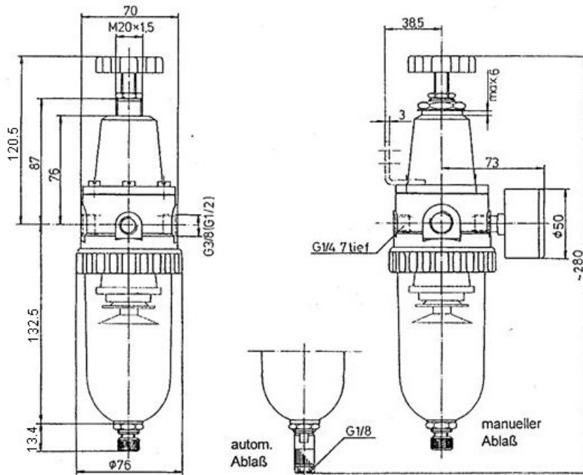
Filterregler mit Polycarbonatbehälter
