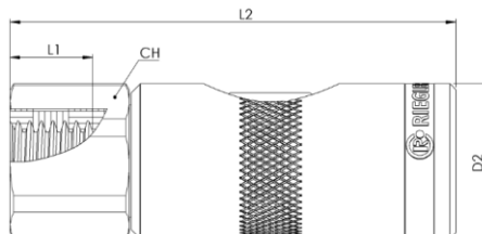
Innengewinde
