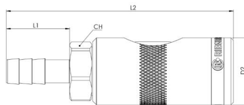
Schlauchtülle
